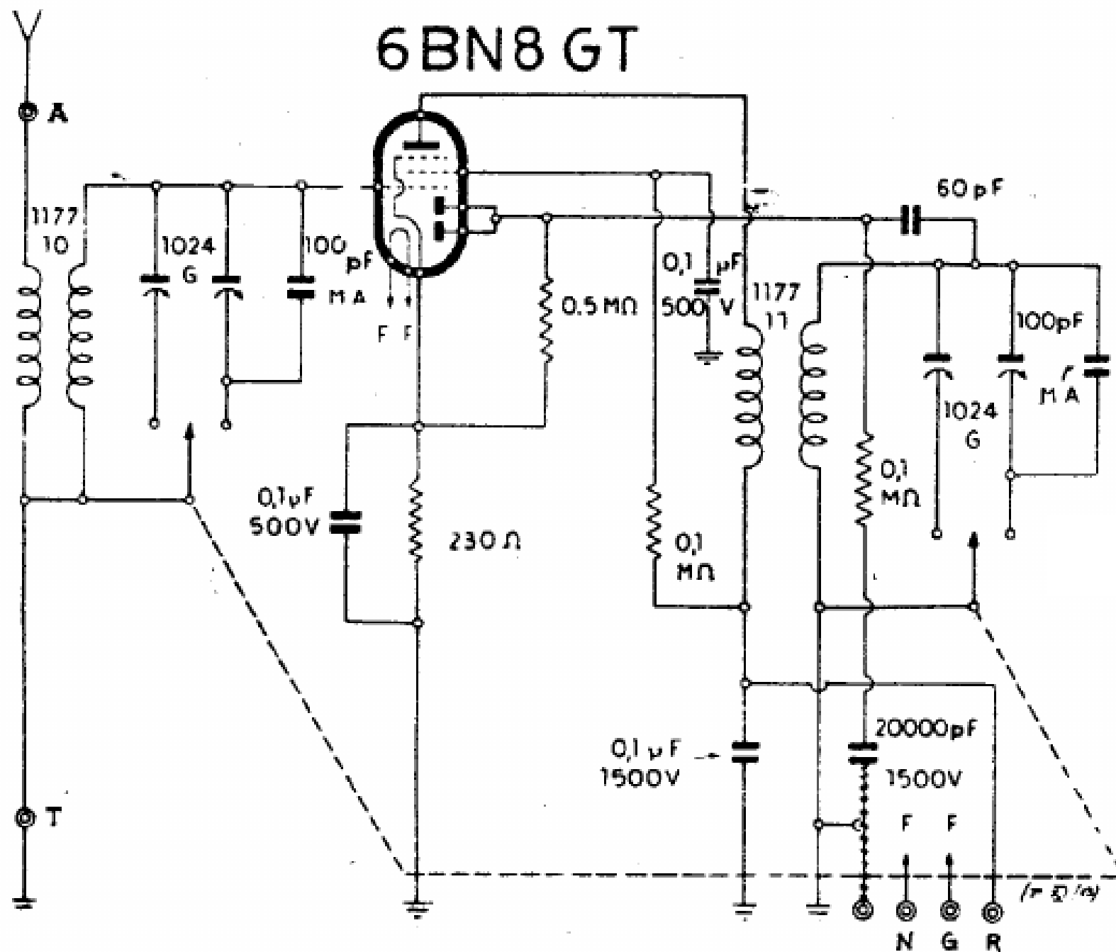
GALLO ING. G. - SINTONIZZATORE CONDOR - MOD. « B »
